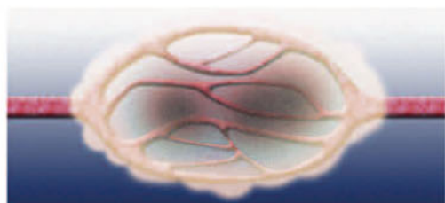
▲がん組織に加温した場合 がん組織は血流が増えないため、熱を逃がすことができず、その結果、血流が減少して温度が上昇し、栄養が行き渡らず死滅に向かう。
